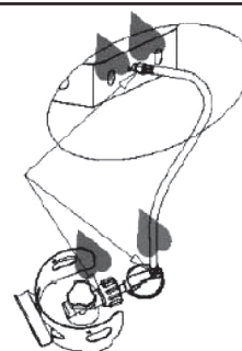
Raccord régulateur-bouteille
